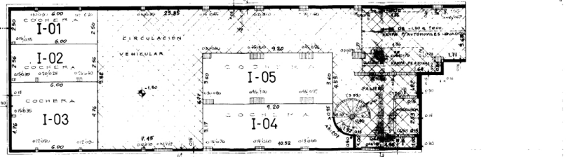
PLANTA SUB-SUELO
