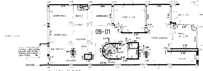
PLANTA 9º PISO
