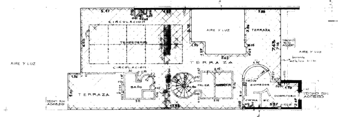
PLANTA DE TERRAZA
