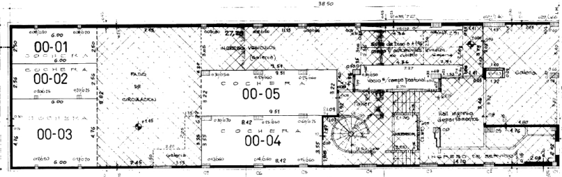
PLANTA BAJA
