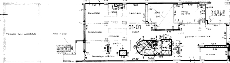
PLANTA 1º PISO
